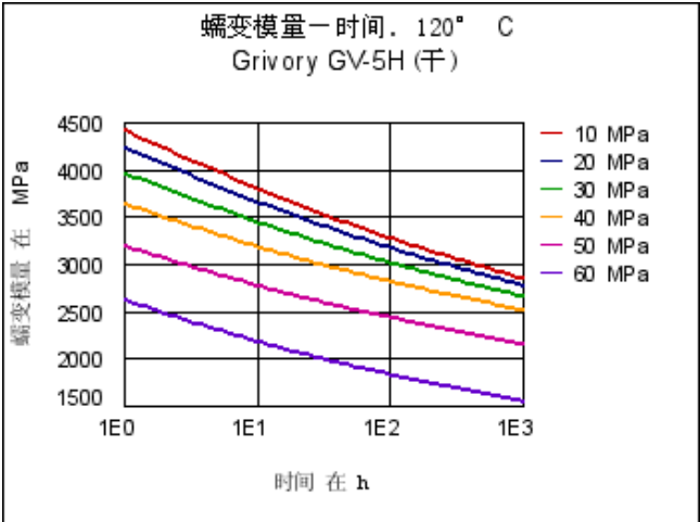
蠕变模量 - 时间. 120 °C
